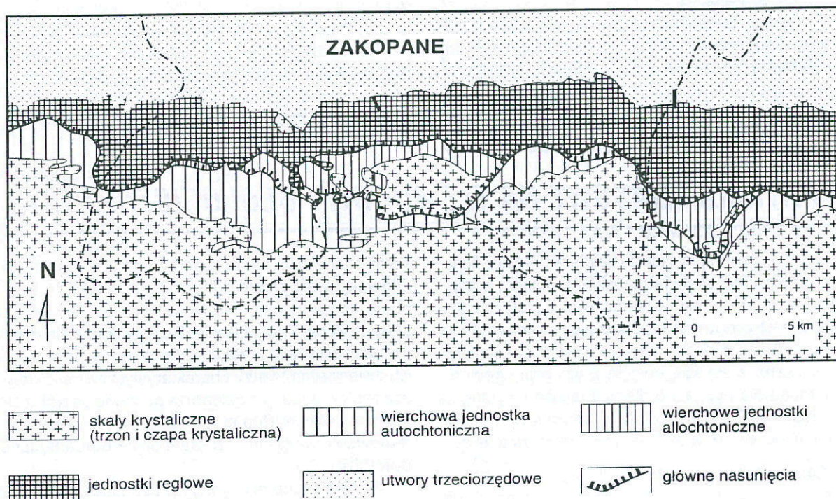
Fig. 1. Schematyczna mapa tektoniczna Tatr (wg Bac-Moszaszwili i in. 1979 - uproszczona)
