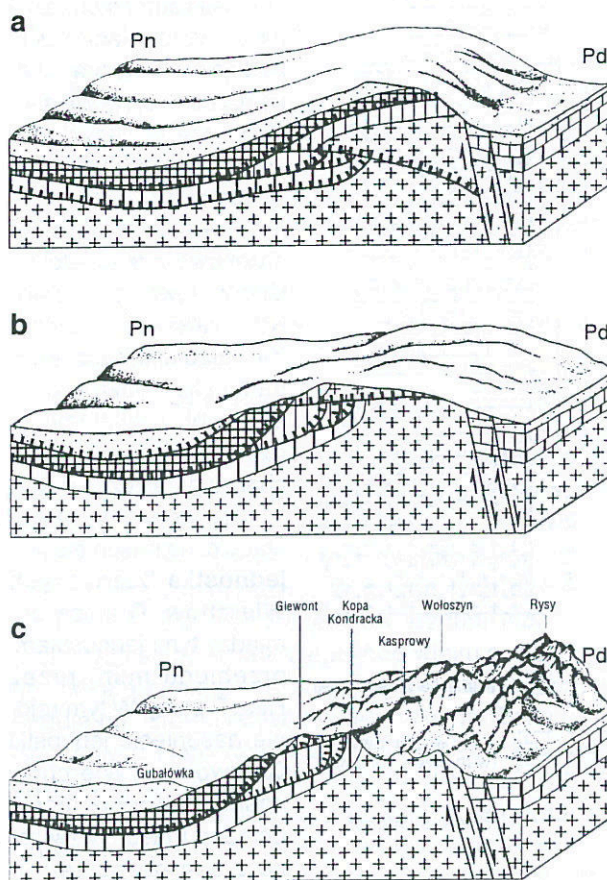
Fig. 5 Przekroje obrazujące podnoszenie Tatr i rozwój rzeźby tatrzańskiej w trzeciorzędzie i czwartorzędzie; a - podnoszenie Tatr w późnym trzeciorzędzie, b-podnoszenie i postępująca erozja na przelomie trzeciorzęd/czwartorzęd, c-sytuacja w czwartorzędzie; oznaczenia jak na Fig. 1 (wg Bac-Moszaszwili i Gąsienica-Szostak, 1990 - zmienione)
